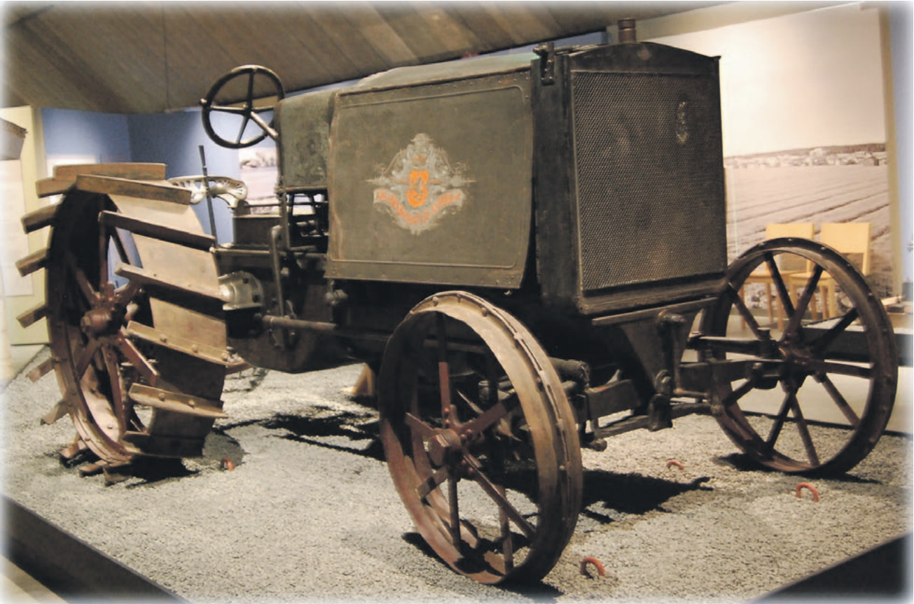
Kullervo-traktori, valmistaja Åbo Jern Manufaktur Aktiebolag. Kuvassa alla Nelipyörärattaat – karjalaiset vankkurit – kärrit – kiesit – rakkaalla lapsella on monta nimeä, vai onko? Miten muistat kotonasi näitä kulkupelejä kutsutun? Kuvan oikeudet: Suomen maatalousmuseo Sarka, jonka esinelistauksista nämä löytyivät nimellä karjalaiset vankkurit.
